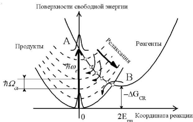
Рис. 1. Неравновесная РЗ в рамках многоканальной стохастической модели. Процесс фотовозбуждения ДАКа под действием импульса накачки с несущей частотой \omega_e изображен вертикальной стрелкой. Волновой пакет, локализованный на терме реагентов (точка А), изображает неравновесное состояние ядерной подсистемы. Пунктиром показаны термы для колебательно-возбужденных состояний продуктов. Движение волнового пакета по поверхности свободной энергии реагентов вдоль координаты реакции от точки А к точке В соответствует релаксации среды. РЗ в точках пересечения термов схематично показана стрелками
