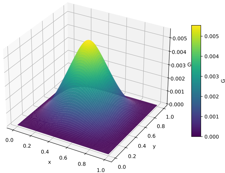
Рис. 2. Функция Грина G_N(\mathbf{r}; (\frac{1}{2}, \frac{1}{2})) бигармонического оператора при источнике в центре квадрата; полиномиальный базис Лежандра, M = 14
