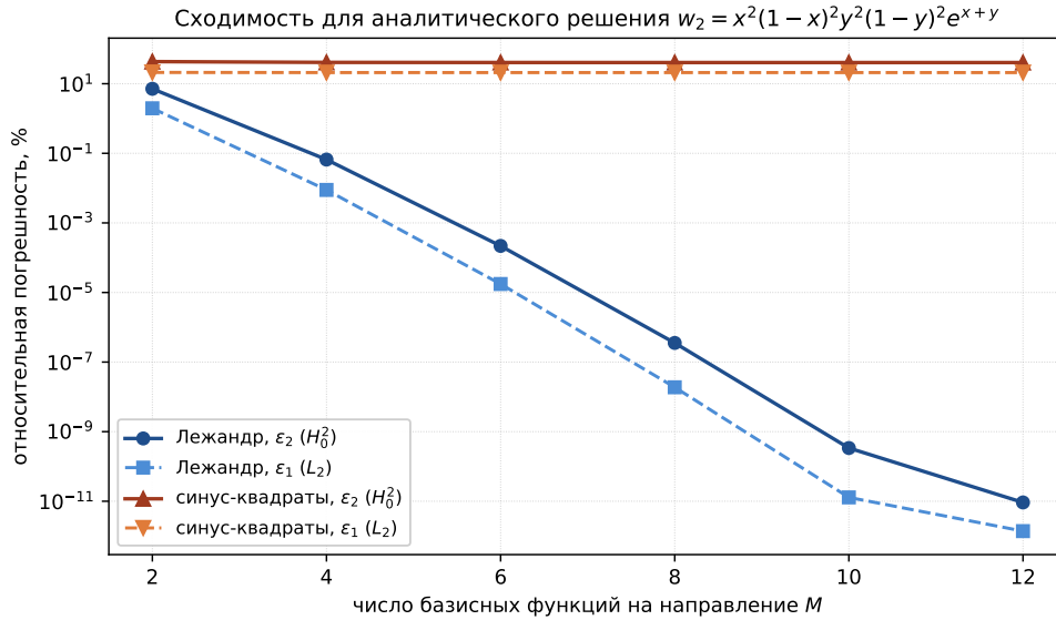
Рис. 1. Сходимость для аналитического решения w_2 : экспоненциальное убывание погрешности полиномиального базиса Лежандра и стагнация тригонометрического базиса синус-квадратов (полулогарифмический масштаб)
