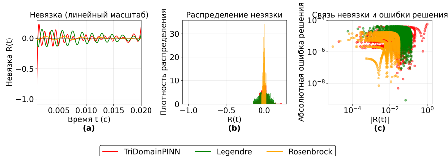
Анализ невязки решений
