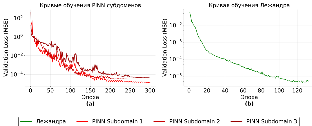
Рис. 7. Кривые обучения TriDomainPINN и Лежандра (8)
