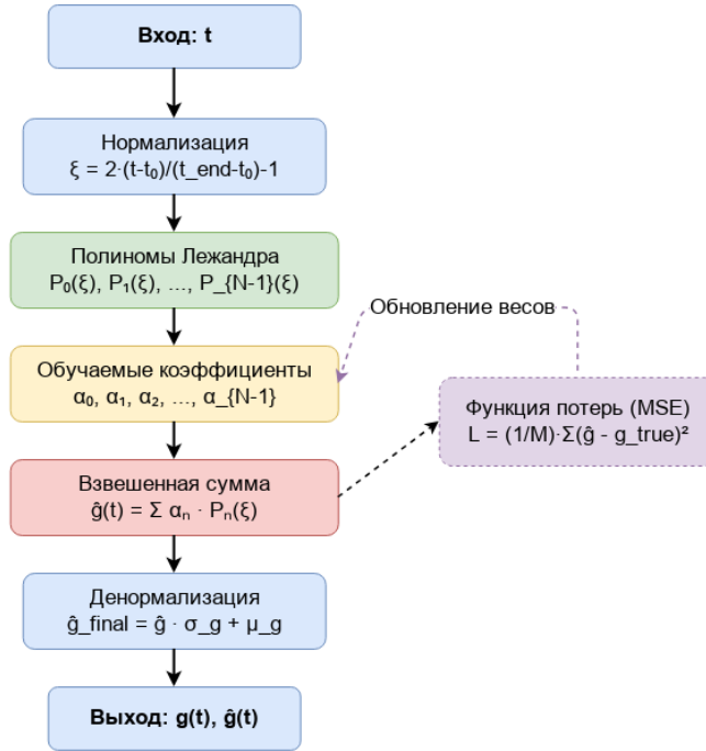
Рис. 5. Архитектура сети LeNN
