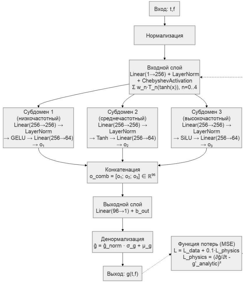
Рис. 3. Архитектура сети TriDomainPINN
