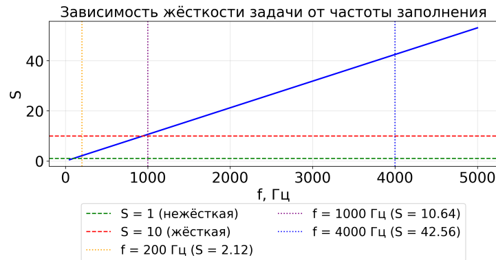
Рис. 2. Зависимость жесткости модели (8) от частоты заполнения f
