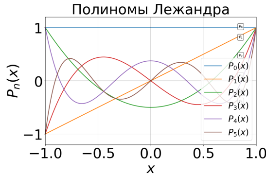
Рис. 4. Полиномы Лежандра
