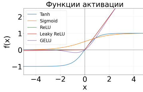
Рис. 6. Функции активации
