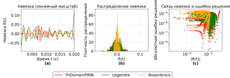
Рис. 8. Анализ невязки решений модели (8). Пример 1
