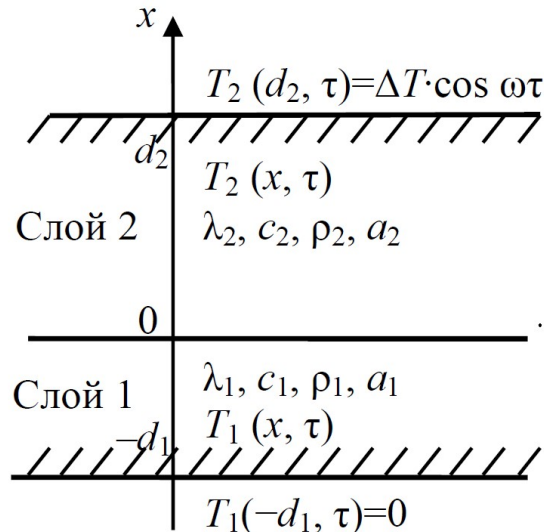
Рис. 1. Постановка задачи о расчете температурного поля в двухслойной пластине
