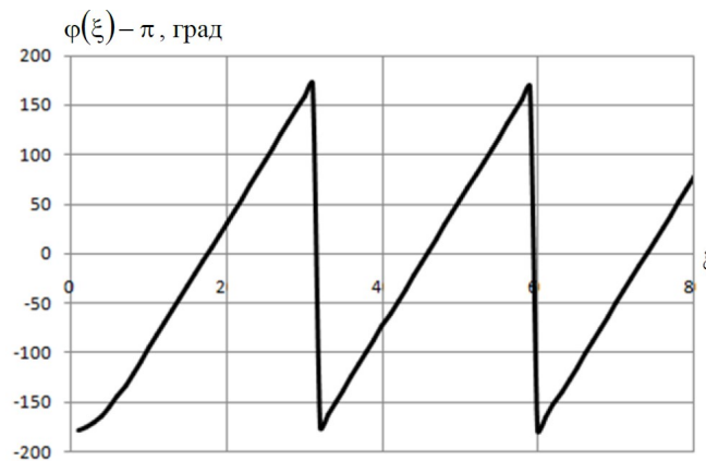
Рис. 3. График аргумента комплексного коэффициента теплопередачи по переменной составляющей
