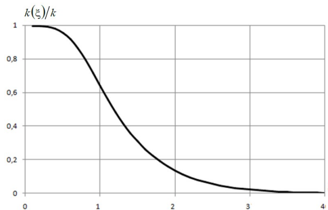
Рис. 2. График модуля коэффициента теплопередачи по переменной составляющей
