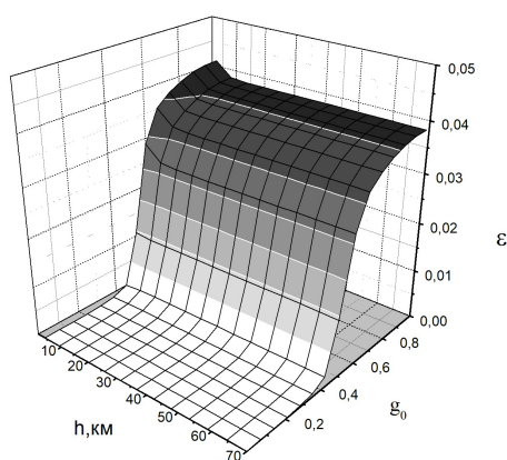
Рис. 4. Погрешность расчета пропускания атмосферы в случае поглощения H_2O и O_3 в спектральном интервале 1060-1080 \text{ см}^{-1} . Функция пропускания на разных атмосферных трассах варьировалась в пределах 0.004-0.9
