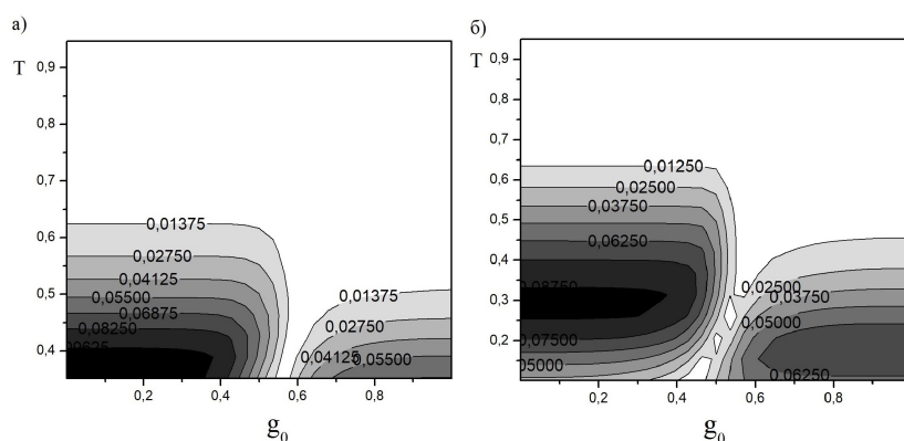
Рис. 6. Погрешность расчета пропускания атмосферы в случае поглощения H_2O и CH_4 в спектральном интервале 2900\text{--}2950\text{ см}^{-1} (а), 2950\text{--}3000\text{ см}^{-1} (б). По оси ординат отложено значение функции пропускания на разных атмосферных трассах от высоты h до 70 км, где h – нижняя граница, которая изменялась 0\text{--}69 км с шагом 1 км
