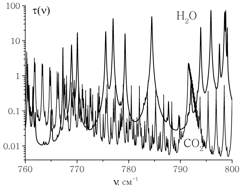
Рис. 1. Фрагмент спектра поглощения \text{H}_2\text{O} и \text{CO}_2 для летних условий метеомодели AFGL [22; 32] для однородной горизонтальной трассы длиной 1 км
