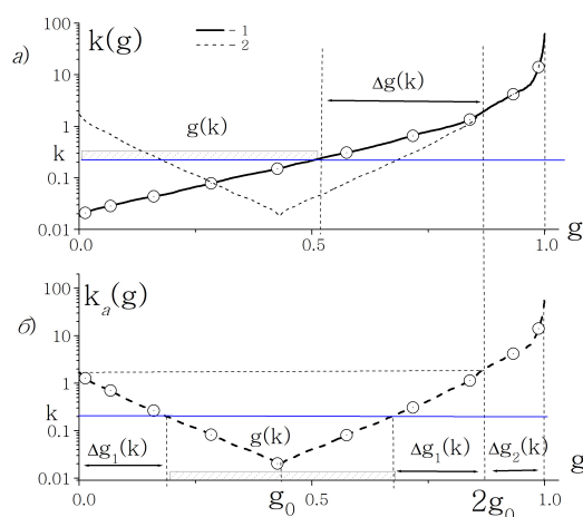
Рис. 3. Методика построения функции k_a(g) (2) (а), 1 - исходная функция k(g) . Кружками обозначены узлы гауссовских квадратур
