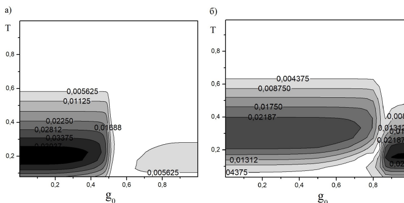
Рис. 7. Погрешность расчета пропускания атмосферы в случае поглощения H_2O и CH_4 в спектральном интервале 2970\text{--}2975\text{ см}^{-1} (а), 2980\text{--}2985\text{ см}^{-1} (б).
