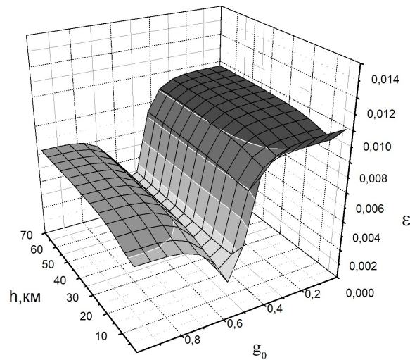
Рис. 5. Погрешность расчета пропускания атмосферы в случае поглощения \text{H}_2\text{O} и \text{CO}_2 в спектральном интервале 760\text{--}800\text{ см}^{-1} . Функция пропускания на разных атмосферных трассах варьировалась в пределах 0.04\text{--}0.9
