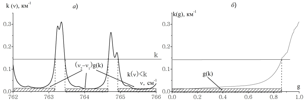
Рис. 2. Фрагмент спектра поглощения \text{H}_2\text{O} . Заштрихованный интервал определяет функцию распределения коэффициента поглощения
