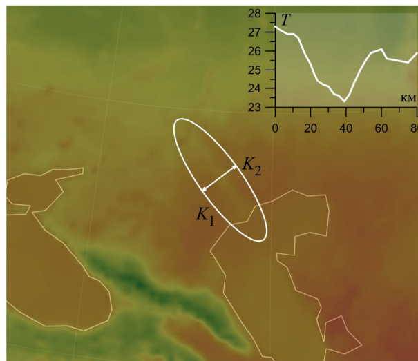
Рис. 9. Охлаждающий эффект от Волго-Ахтубинской поймы, наблюдаемый 07.07.2019.
