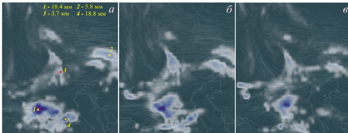
Рис. 12. Распределения осадков по данным earth.nullschool.net (система координат отличается от используемой на рисунке 11)
