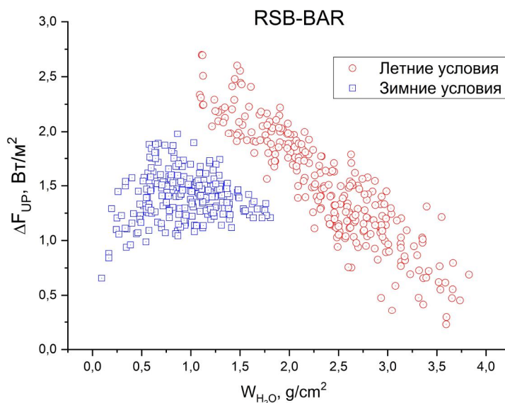
Рис. 4. Расхождения в восходящих потоках излучения на верхней границе атмосферы при использовании модели континуума RSB и модели BAR
