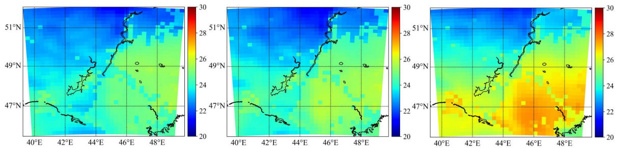
Рис. 8. Зависимость температуры T в области D для моделей A, B, C (слева–направо) для июня 2016 года по результатам нашего моделирования
