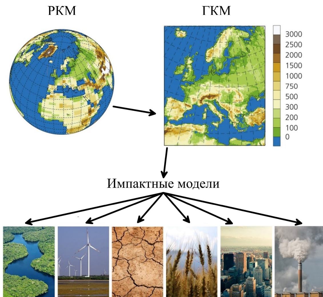
Рис. 1. Области приложений региональных климатических моделей
