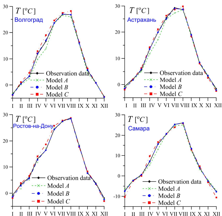
Рис. 7. Зависимость температуры T от времени в течение 2016 года для четырех городов: Волгоград, Астрахань, Ростов-на-Дону, Самара
