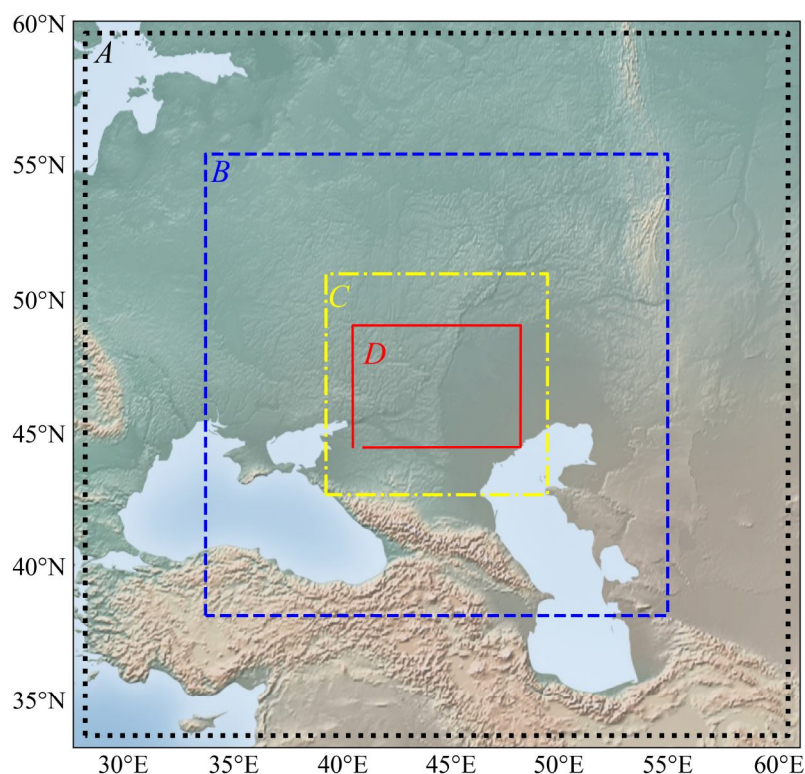
Рис. 6. Различные вычислительные области, используемые для моделирования: A — базовая модель размером 2000 \times 2000 км с центром в г. Волгоград, модели B , C , D имеют меньшую площадь
