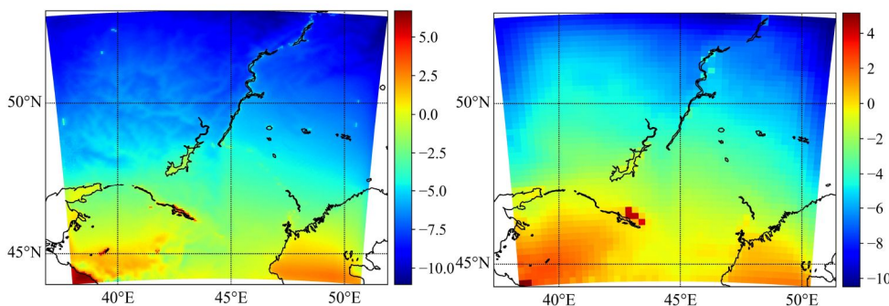
Рис. 10. Сравнение среднемесячного распределения температуры января 2016 для негидростатического (слева) и гидростатического (справа) ядер
