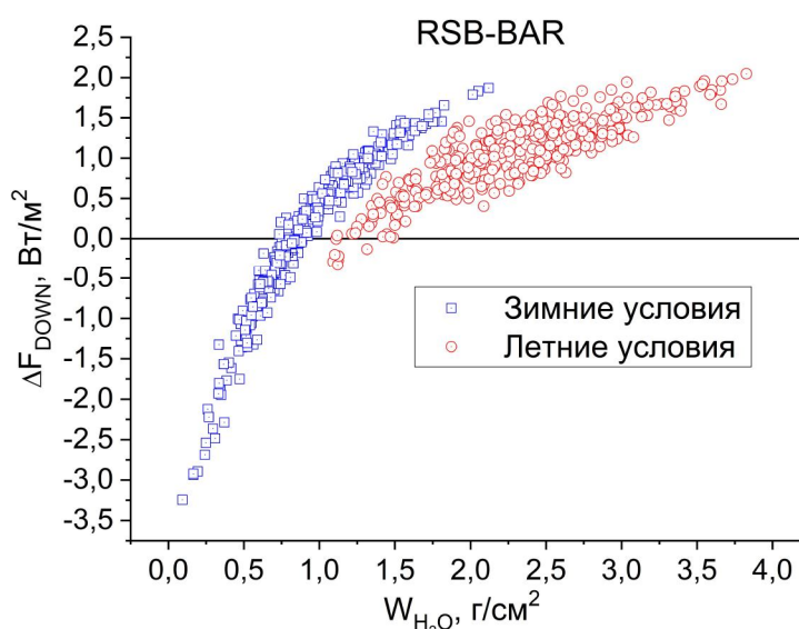
Рис. 5. Расхождения в нисходящих потоках излучения на нижней границе атмосферы при использовании модели континуума RSB и модели BAR
