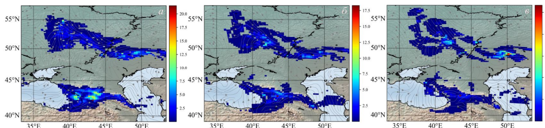
Рис. 11. Результаты климатического моделирования: распределения осадков
