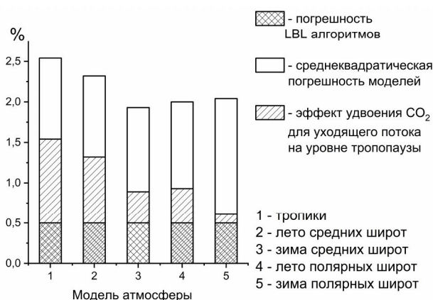
Рис. 3. Сравнение СКО потоков восходящей длинноволновой радиации на уровне тропопаузы, которые рассчитаны приближенными и прямыми методами, а также радиационный форсинг, обусловленный удвоением концентрации \text{CO}_2
