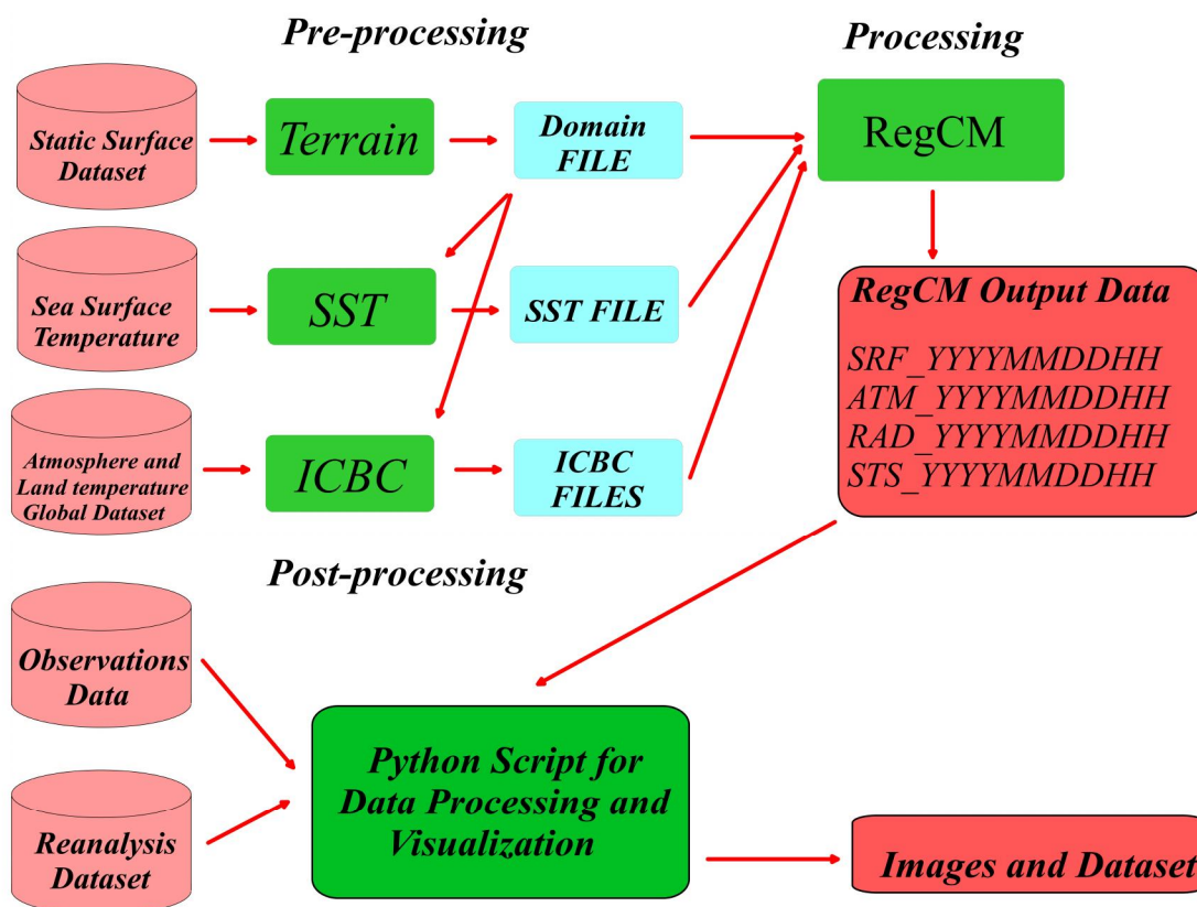
Рис. 2. Схема работы с моделью RegCM
